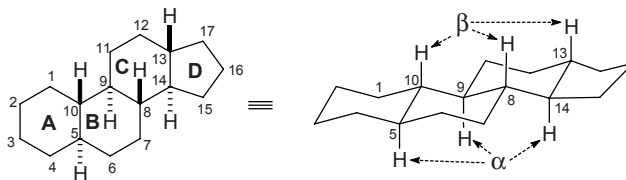
A/B trans : 5\alpha -Steran (ausgewählte \alpha - und \beta -Positionen sind markiert)
