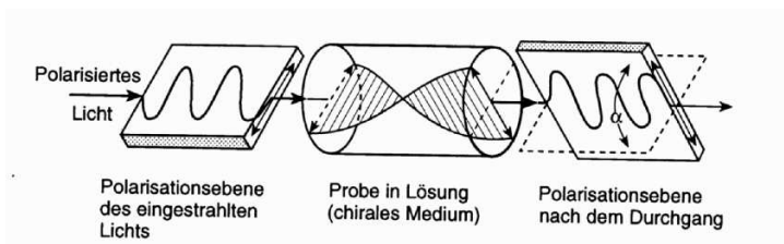
Abb. 58. Polarimeter (schematisch)
