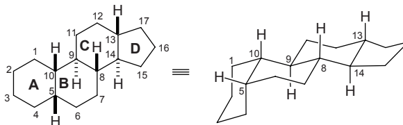
A/B trans : 5\alpha -Steran (ausgewählte \alpha - und \beta -Positionen sind markiert)
