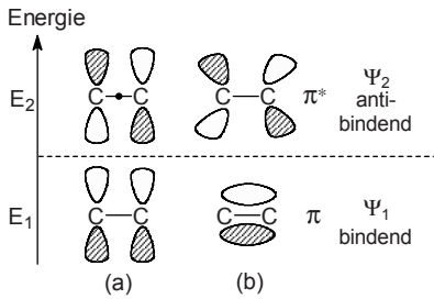
Abb. 24. a Basis-AO der \pi -MO im Ethen. b die delokalisierten \pi -MO
