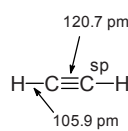
Ethin
