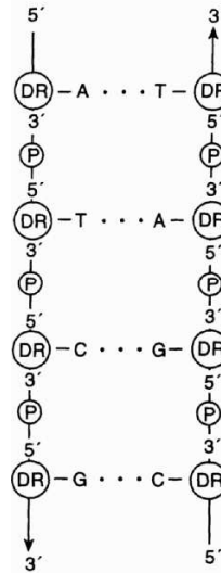
Abb. 78. Anordnung komplementärer DNA-Stränge in Gegenrichtung DR = Desoxyribose
