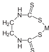
Maneb für M = \text{Mn}
