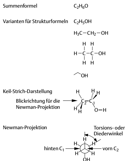
Abb. 3.13 Verschiedene Darstellungsmöglichkeiten für Ethanol
