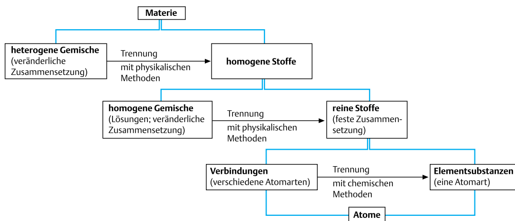
Abb. 1.2 Einteilung der stofflichen Materie
