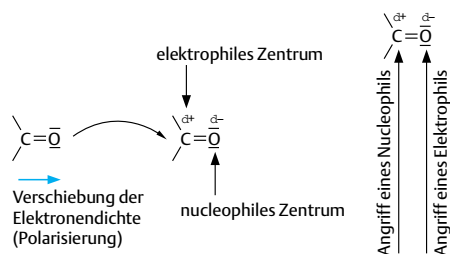
Abb. 4.29 Die Polarisierung der Carbonylgruppe und die reaktiven Zentren
