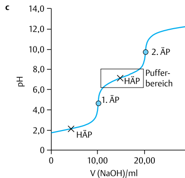
Abb. 2.15 Titrationskurven für die Titration verschiedener Säuren mit Natronlauge; (a) Titration von Salzsäure (HCl) mit NaOH; (b) Titration von Essigsäure ( \text{CH}_3\text{COOH} ) mit NaOH; (c) Titration von Phosphorsäure ( \text{H}_3\text{PO}_4 ) mit NaOH
