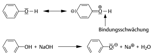
Abb. 4.13 Phenol als Protonendonator
