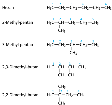
Abb. 3.21 Isomere mit der Summenformel C_6H_{14}
