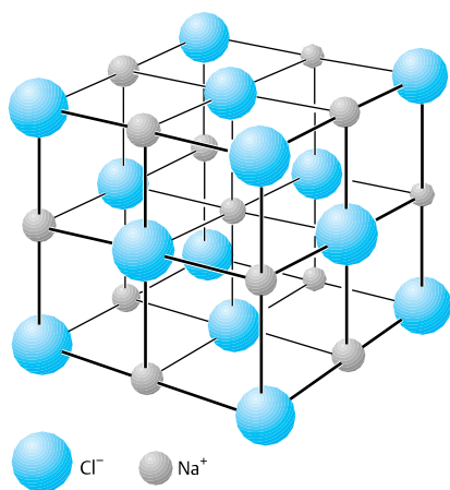
Abb. 1.13 Schematische Darstellung des Natriumchloridgitters
