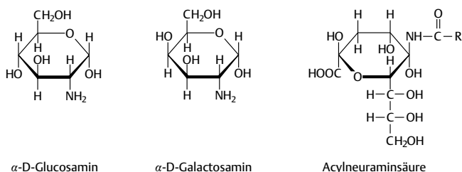
Abb. 5.22 Weitere biochemisch wichtige Monosaccharide
