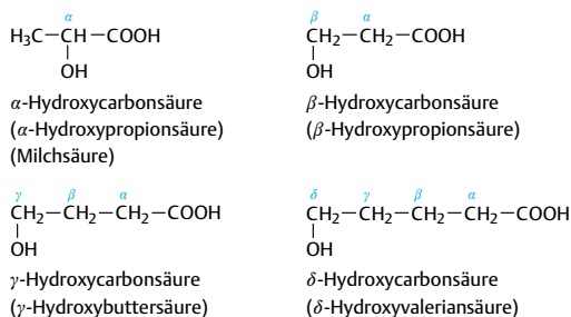
Abb. 3.18 Nummerierung der Kohlenstoffatome mit griechischen Buchstaben
