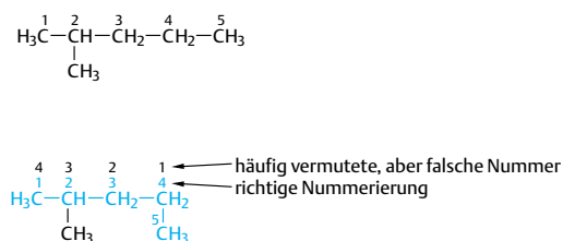
Abb. 3.22 2-Methyl-pentan (nicht 1,3-Dimethylbutan)
