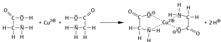
Abb. 5.6 Die Aminosäuren als zweizählige Liganden
