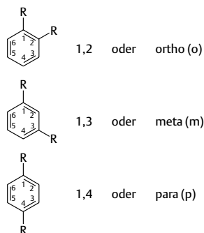
Abb. 3.17 Stellung der Substituenten bei cyclischen Kohlenwasserstoffen
