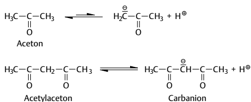
Abb. 4.37 C-H-Azidität von Aceton und Acetylaceton
