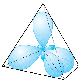
Abb. 3.2 Optimale Anordnung der sp 3 -Hybridorbitale
