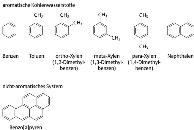
Abb. 4.7 Aromatische Kohlenwasserstoffe und Benzo[a]pyren
