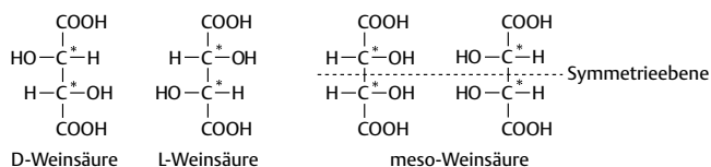
Abb. 3.43 Stereoisomere der Weinsäure
