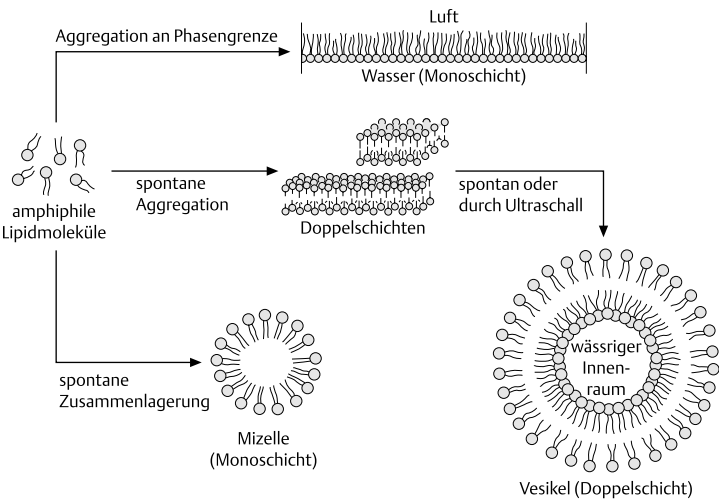
Abb. 5.33 Die Zusammenlagerung von Lipidmolekülen
