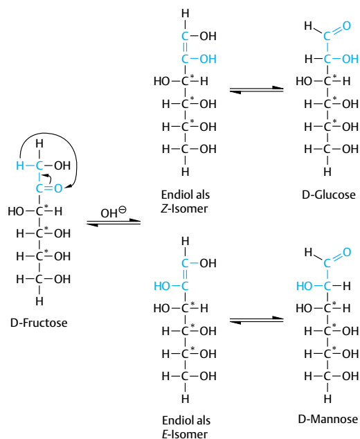
Abb. 5.20 Die Tautomerie bei Fructose
