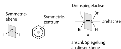
Abb. 3.33 Symmetrieebene, Symmetriezentrum und Drehspiegelachse
