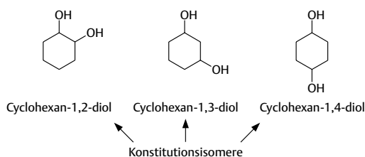
Abb. 3.29 Die konstitutionsisomeren Cyclohexandiole
