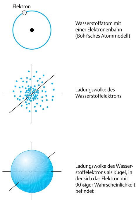
Abb. 1.6 Verschiedene Darstellungen des Elektrons eines Wasserstoffatoms im Grundzustand
