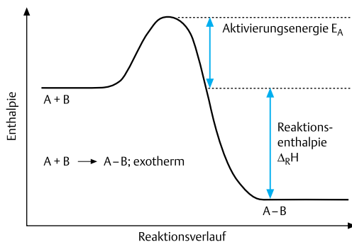
Abb. 2.9 Die Aktivierungsenergie und die Änderung der Reaktionsenthalpie im Reaktionsverlauf
