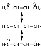
Abb. 3.9 Mesomere Grenzstrukturen von Buta-1,4-dien
