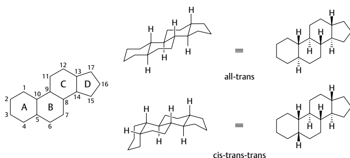
Abb. 5.35 Gonan mit Nummerierung und Bezeichnung der Ringe sowie all-trans und cis-trans-Verknüpfung der Ringe A und B
