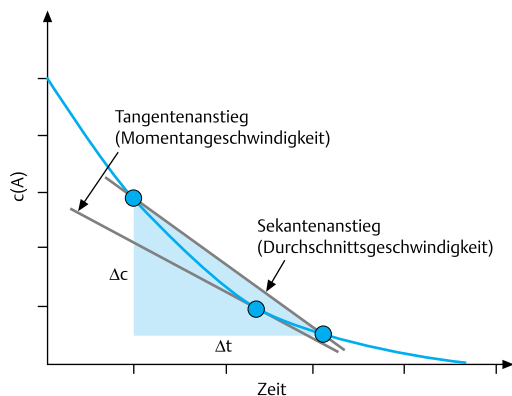
Abb. 2.7 Die Momentan- und die Durchschnittsgeschwindigkeit
