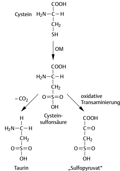
Abb. 4.18 Die kräftige Oxidation von Cystein und Folgereaktionen (OM = Oxidationsmittel)
