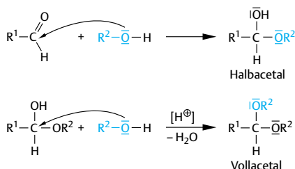
Abb. 4.33 Die Bildung von Halb- und Vollacetalen
