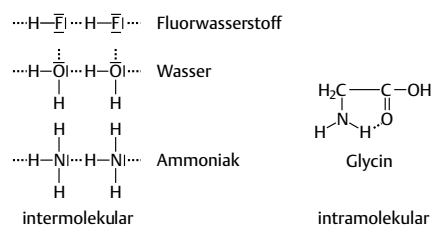
Abb. 1.18 Wasserstoffbrückenbindungen
