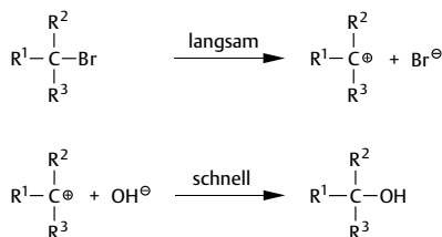
Abb. 3.55 Die nucleophile Substitution nach einem S_N^1 -Mechanismus
