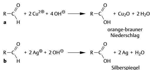
Abb. 5.19 Fehlingsche Lösung (a) und Tollens-Reagens (b) als Oxidationsmittel
