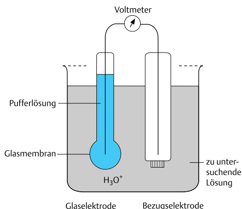
Abb. 2.24 Die schematische Anordnung zur Messung des pH-Wertes mit einer Glaselektrode
