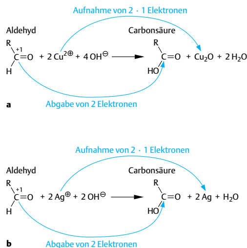
Abb. 4.40 Reaktion eines Aldehyds mit Fehlingscher Lösung (a) und Tollens-Reagens (b)
