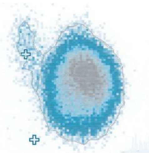
Abb. 1.4 Szintigramm der Schilddrüse nach Injektion von ^{99m}_{43}\text{Tc} (Adenom linksseitig)
