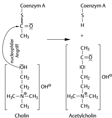
Abb. 4.46 Acetyl-Coenzym A als Acetylgruppenüberträger
