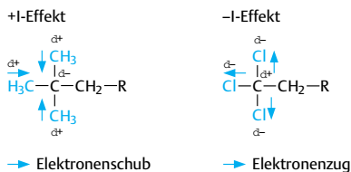
Abb. 3.48 Der induktive Effekt
