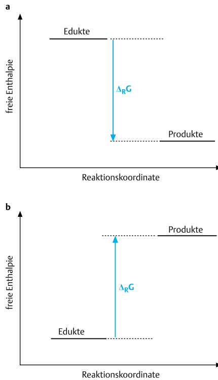
Abb. 2.2 Die Änderung der freien Enthalpie bei einer exergonen (a) und einer endergonen (b) Reaktion
