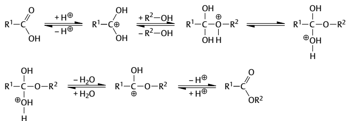
Abb. 4.47 Schema der Veresterung („Hinreaktion“) und der Esterhydrolyse („Rückreaktion“)
