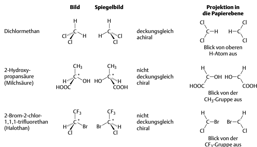
Abb. 3.32 Achirale und chirale Moleküle
