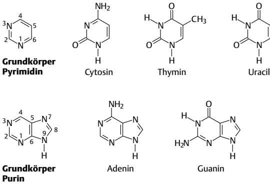
Abb. 5.38 Purin- und Pyrimidinbasen
