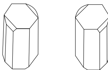
Abb. 3.31 Spiegelbildliche Kristalle der Natrium-Ammonium-Tartrate
