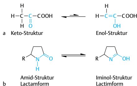
Abb. 3.57 Keto-Enol-Tautomerie bei Brenztraubensäure (a), Lactam-Lactim-Tautomerie bei einem ringförmigen Amid (b)
