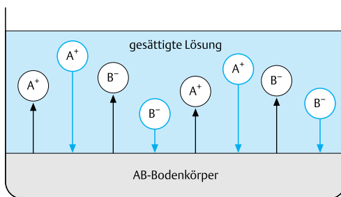
Abb. 2.13 Schematische Darstellung des Gleichgewichts in einer gesättigten Salzlösung
