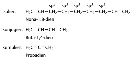
Abb. 3.7 Isolierte, konjugierte und kumulierte Doppelbindungen
