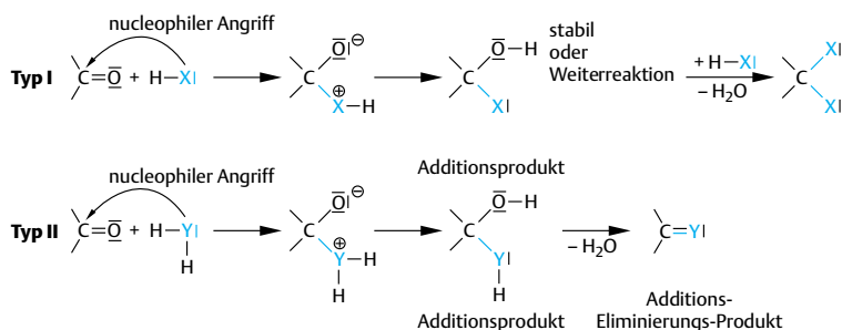
Abb. 4.30 Schema des Angriffs eines Nucleophils
