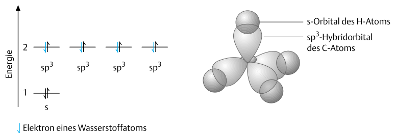
Abb. 3.4 Das Energieniveauschema und die Orbitaldarstellung für Methan
