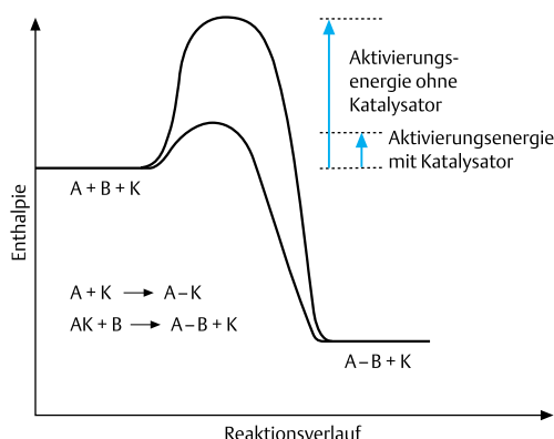
Abb. 2.10 Vergleich der Energiediagramme einer Reaktion mit und einer Reaktion ohne Katalysator
