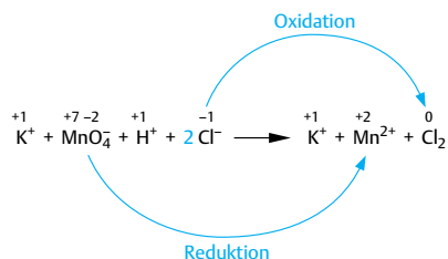
Abb. 2.18 Kennzeichnen der Oxidation und der Reduktion
