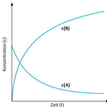
Abb. 2.6 Die Veränderung der Konzentration ( c ) in Abhängigkeit von der Zeit ( t )
