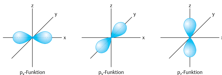
Abb. 1.7 Die räumliche Darstellung der p-Orbitale
