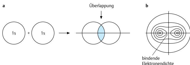
Abb. 1.15 Die Überlappung der s-Orbitale zweier Wasserstoffatome (a) und die Darstellung der Elektronendichte im Wasserstoffmolekül (b)
