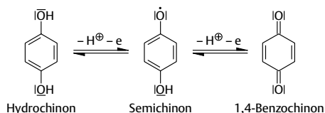
Abb. 4.14 Oxidation von Hydrochinon
