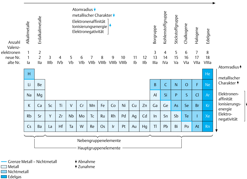
Abb. 1.10 Der Aufbau und die Gesetzmäßigkeiten im PSE
