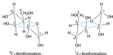
Abb. 5.16 Die Sesselschreibweisen der \alpha -D-Glucopyranose
