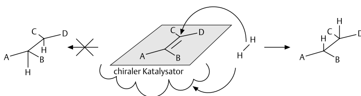
Abb. 3.40 Enantioselektive Hydrierung
