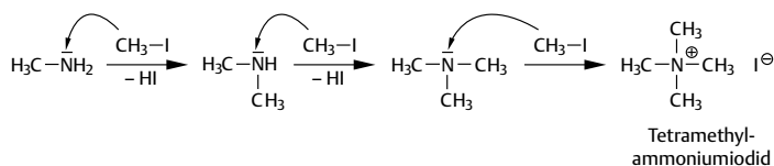
Abb. 4.25 Die vollständige Alkylierung von Methylamin (HI = Iodwasserstoff, \text{CH}_3-\text{I} = Methyljodid)
