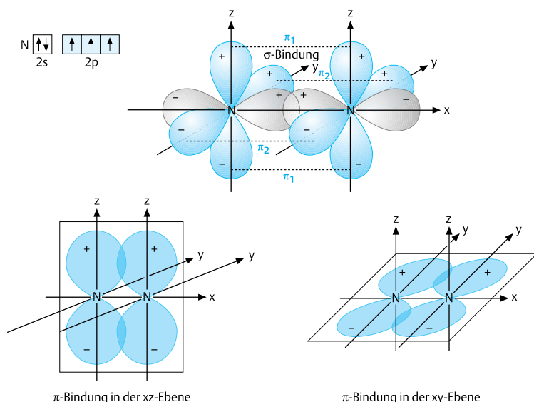
Abb. 1.16 Die Elektronenkonfiguration des Stickstoffatoms und die Überlappung der p-Orbitale des Stickstoffmoleküls
