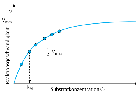
Abb. 2.11 Die Abhängigkeit der Reaktionsgeschwindigkeit einer enzymkatalysierten Reaktion von der Substratkonzentration
