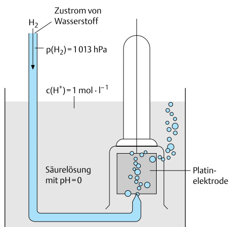
Abb. 2.22 Der Aufbau der Standardwasserstoffelektrode
