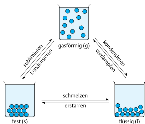
Abb. 1.1 Die Änderungen des Aggregatzustands
