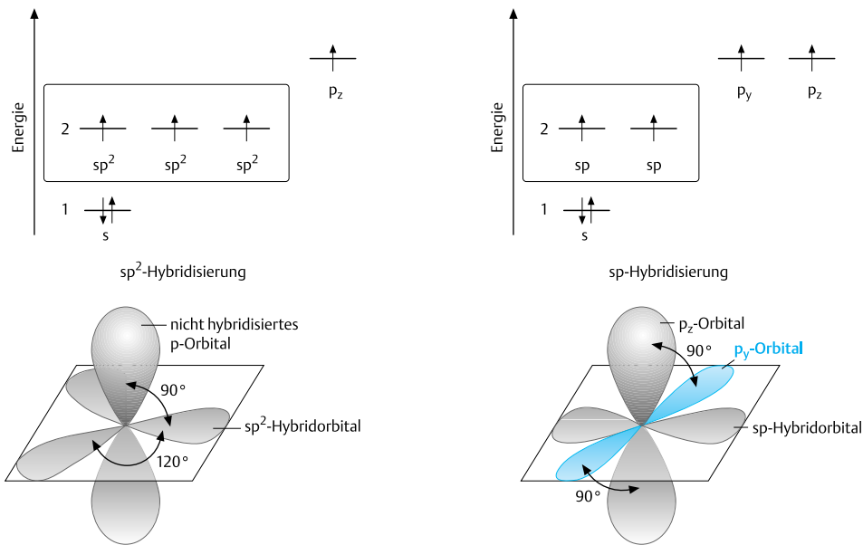
Abb. 3.3 Die Elektronenkonfiguration für die sp^2 - und sp -Hybridisierung sowie die räumliche Darstellung der Orbitale
