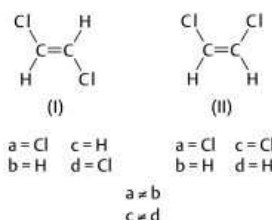
Abb. 3.24 Isomere des 1,2-Dichlorethans
