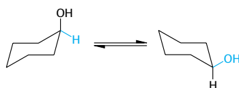
Abb. 3.28 Die alternativen Sesselformen des Cyclohexanols
