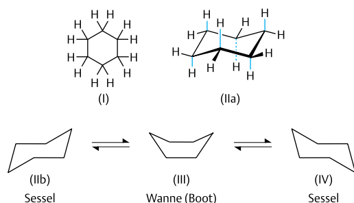
Abb. 3.27 Die Konformeren des Cyclohexans
