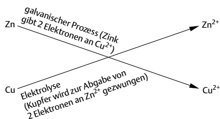
Abb. 2.25 Der galvanische Prozess und die Elektrolyse im Daniell-Element
