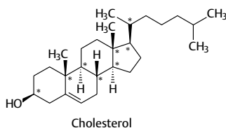
Abb. 5.36 Struktur des Cholesterols
