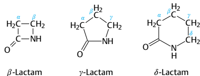
Abb. 4.51 Cyclische Carbonsäureamide
