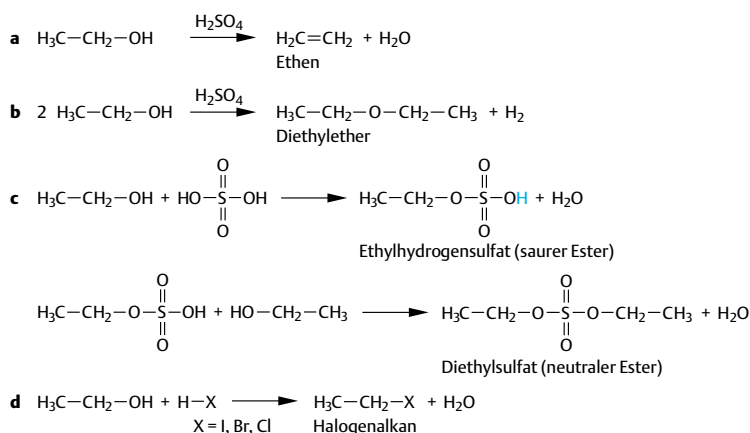
Abb. 4.10 Die Reaktionen von Ethanol mit Schwefelsäure (a–c) und mit Halogenwasserstoffsäuren (d)
