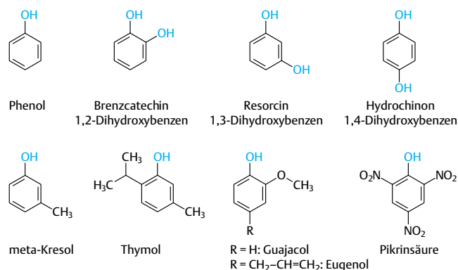
Abb. 4.12 Einige Beispiele für Phenole
