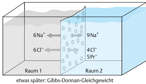
Abb. 2.29 Das Gibbs-Donnan-Gleichgewicht hat sich eingestellt
