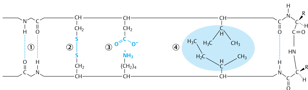
Abb. 5.11 Die Bindungen zwischen verschiedenen Abschnitten der Peptidkette (1 = Wasserstoffbrückenbindung; 2 = Disulfidbrücke; 3 = Ionenbeziehung; 4 = hydrophobe Wechselwirkung, d.h. aus dem blauen Bereich wird Wasser herausgedrängt)
