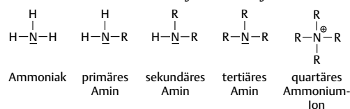
Abb. 4.23 Die Einteilung in primäre, sekundäre, tertiäre Amine und quartäre Ammonium-Ionen
