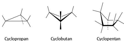
Abb. 4.2 Die Pitzer-Spannung in Ringsystemen
