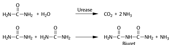
Abb. 4.53 Die enzymatische Spaltung von Harnstoff und die Biuretbildung
