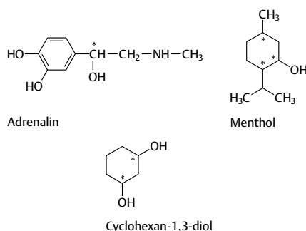
Abb. 3.35 Moleküle mit stereogenen Zentren * (asymmetrisch substituierten C-Atomen)
