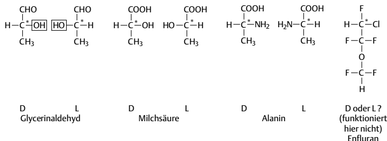
Abb. 3.38 Beispiele für die D/L-Nomenklatur
