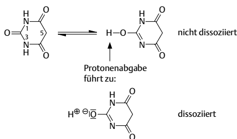
Abb. 3.58 Lactam-Lactim-Tautomerie bei der Barbitursäure
