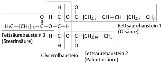
Abb. 5.28 Struktur eines Triglycerids
