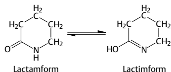
Abb. 4.52 Lactam-Lactim-Tautomerie
