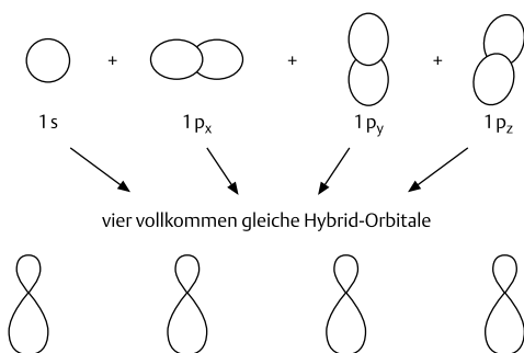
Abb. 3.1 Die Elektronenkonfiguration des Kohlenstoffatoms vor und nach der Hybridisierung und die räumliche Darstellung der Orbitale
