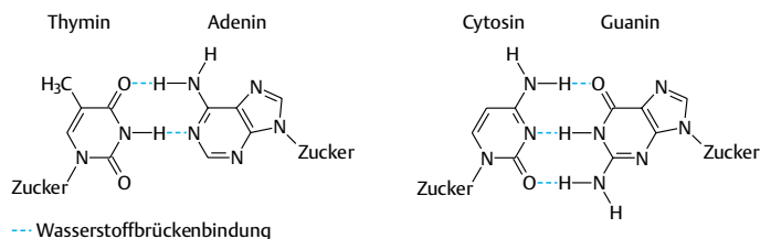
Abb. 5.41 Die Struktur von Desoxyribonukleinsäure (DNA) (a) und Ribonukleinsäure (RNA) (b)
