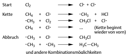
Abb. 3.52 Der radikalische Kettenmechanismus
