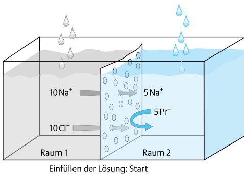
Abb. 2.28 Vor der Ausbildung des Gibbs-Donnan-Gleichgewichts ( \text{Pr}^- = Proteinat)
