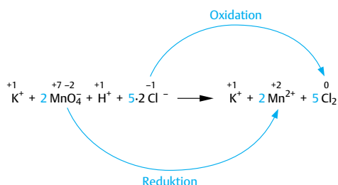
Abb. 2.20 Ausgleich der Elektronenbilanz
