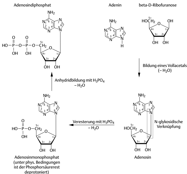
Abb. 5.40 Die Bildung von Adenosin, Adenosinmono- und Adenosindiphosphat
