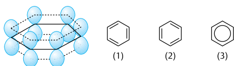
Abb. 3.10 Die nicht hybridisierten p-Orbitale und deren Wechselwirkung sowie die verschiedenen Formelschreibweisen für Benzen
