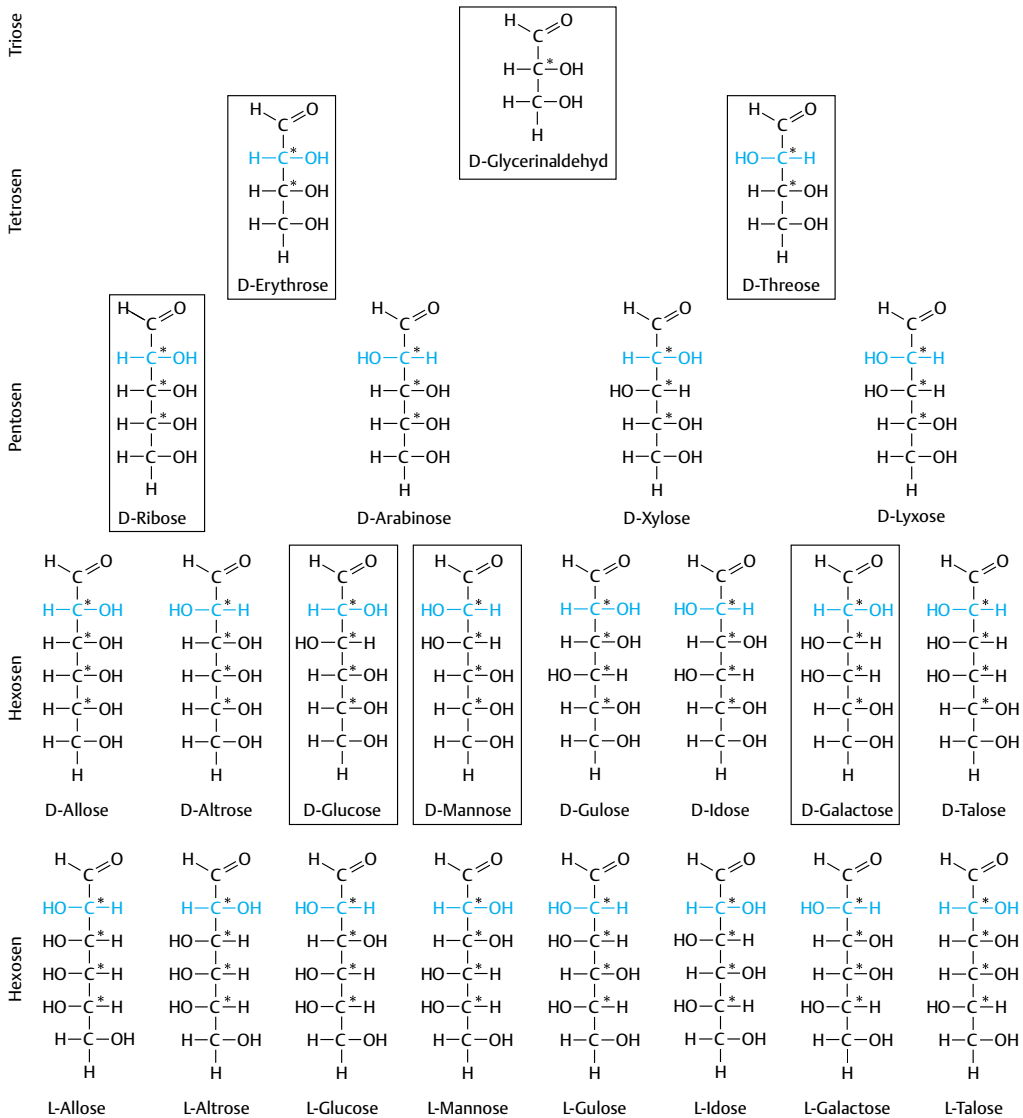
Abb. 5.13 Der Stammbaum der D-Aldosen und die L-Aldohexosen (* = stereogenes Zentrum)
