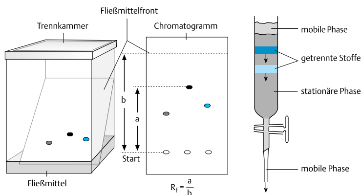
Abb. 3.45 Dünnschicht- und Säulenchromatografie
