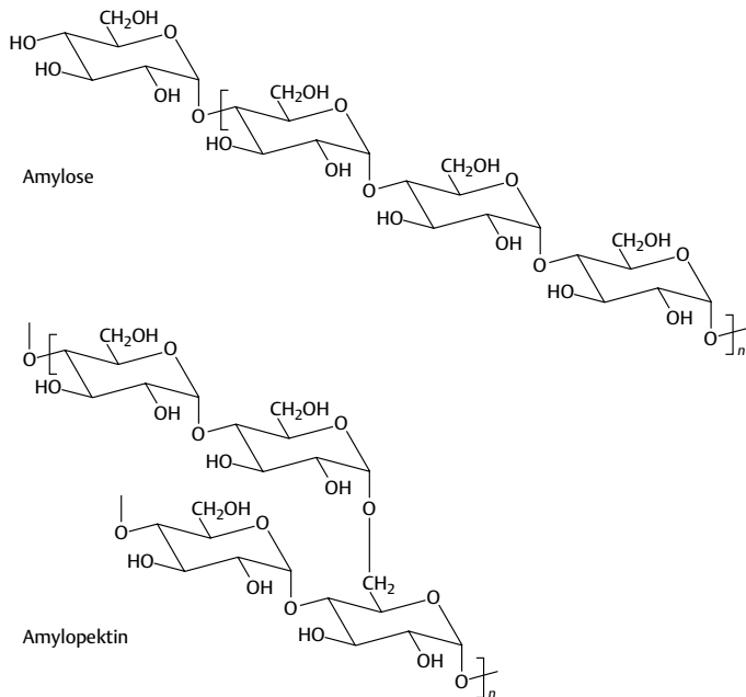
Abb. 5.25 Formelausschnitte Amylose und Amylopektin
