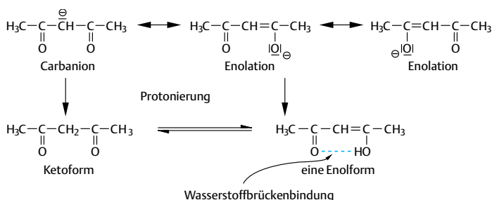
Abb. 4.39 Mesomere und tautomere Formen bei Dicarbonylverbindungen
