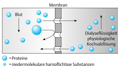
Abb. 2.27 Die schematische Darstellung einer Dialyse
