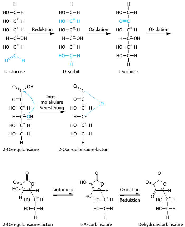
Abb. 5.21 Die vereinfacht formulierte Bildung von L-Ascorbinsäure
