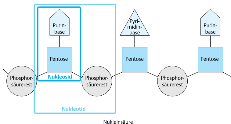
Abb. 5.37 Der schematische Aufbau der Nukleinsäuren
