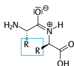
Abb. 5.9 Die Mesomerie und E/Z-Isomerie der Peptidbindung
