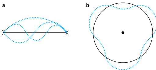
Abb. 1.5 Die Eigenschwingungen einer Saite (a) und die schematisierte Eigenschwingung einer Elektronenwelle auf einer Kreisbahn (b)
