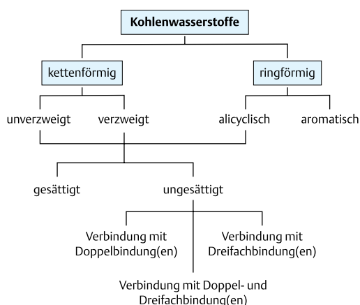
Abb. 3.12 Klassifizierung der Kohlenwasserstoffe und Stoffbeispiele für die einzelnen Klassen
