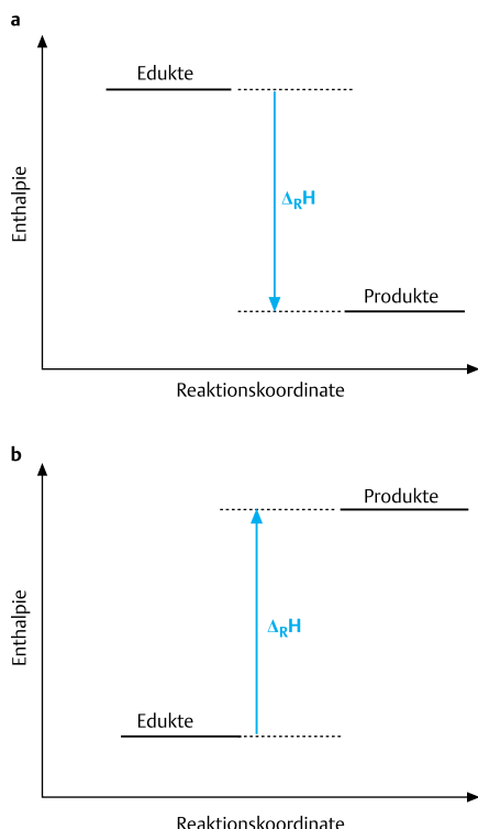
Abb. 2.1 Die Enthalpieänderung bei einer exothermen (a) und einer endothermen (b) Reaktion
