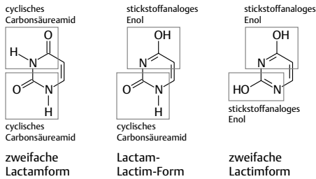
Abb. 5.39 Lactam-Lactim-Tautomerie am Beispiel des Uracil
