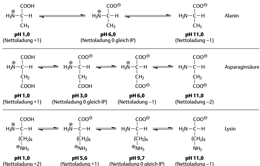
Abb. 5.4 Die Struktur von Alanin, Asparaginsäure und Lysin bei verschiedenen pH-Werten und ihre jeweiligen Nettoladungen
