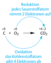
Abb. 2.17 Kennzeichnen der Oxidation und Reduktion
