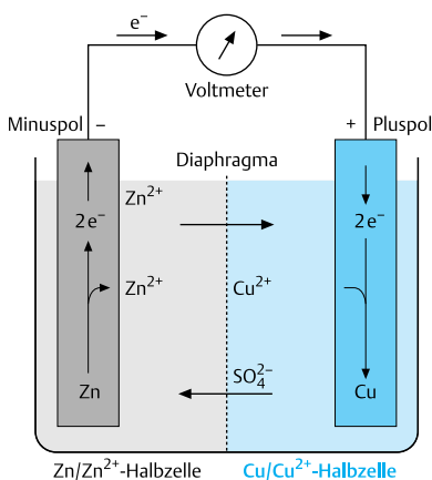
Abb. 2.21 Der schematische Aufbau des Daniell-Elements
