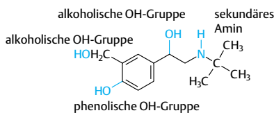
Abb. 3.19 Struktur von Salbutamol (Broncholytikum) und Zuordnung der vier funktionellen Gruppen
