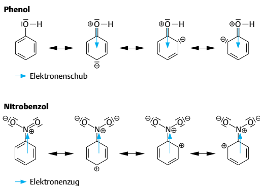
Abb. 3.49 Der mesomere Effekt
