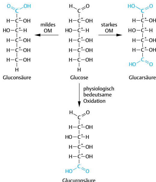
Abb. 5.18 Die Möglichkeiten der Oxidation von D-Glucose (OM=Oxidationsmittel)
