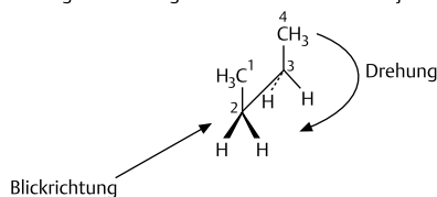
Abb. 3.26 Newman-Projektionen der Konformere des Butans und Energieinhalte
