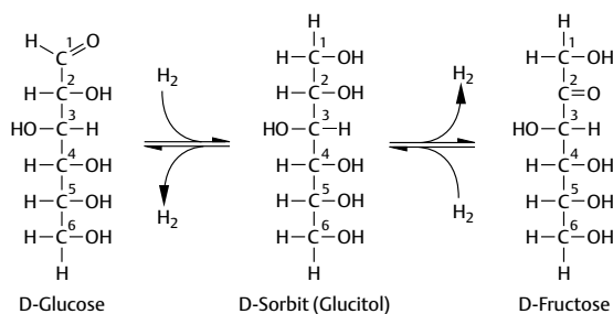
Abb. 5.17 Die Reduktion von Glucose und Fructose zu Sorbit
