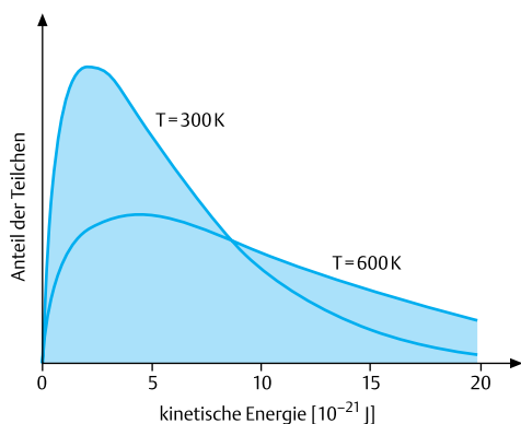
Abb. 2.8 Die Energieverteilung der Teilchen nach Boltzmann für verschiedene Temperaturen ( T = Temperatur)
