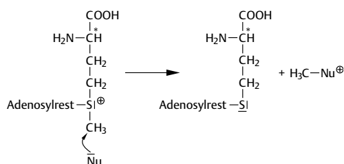
Abb. 4.20 S-Adenosylmethionin als Methylgruppenüberträger (Nu = Nucleophil)
