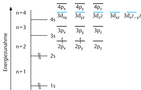
Abb. 1.9 Energieebenauschema für ein System mit 6 Elektronen
