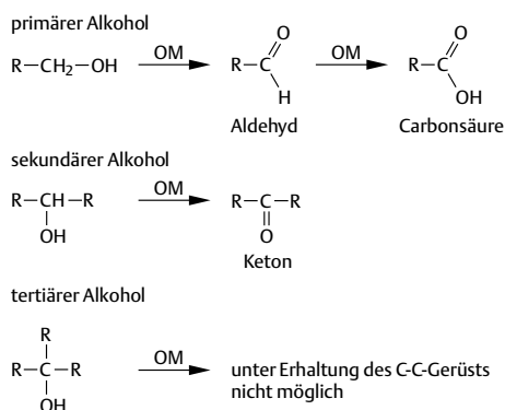
Abb. 4.11 Die Oxidation der Alkohole (OM = Oxidationsmittel)
