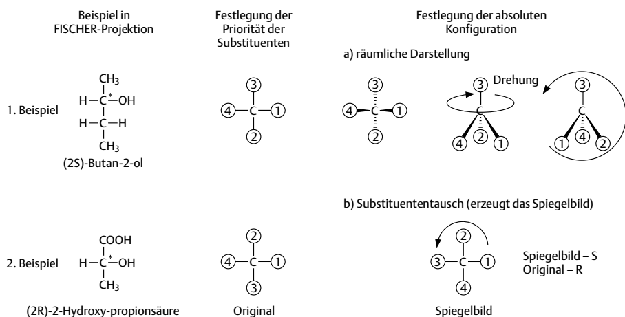
Abb. 3.39 Festlegung der Priorität der Substituenten und Bestimmung der absoluten Konfiguration
