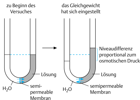
Abb. 2.26 Die schematische Versuchsanordnung zur Osmose
