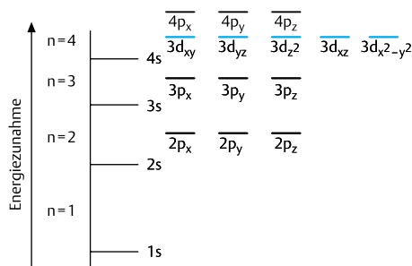
Abb. 1.8 Die verschiedenen Energieebenen
