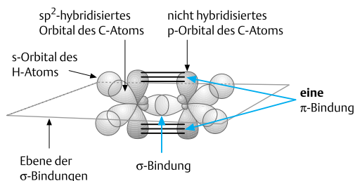
Abb. 3.6 Orbitaldarstellung im Ethen
