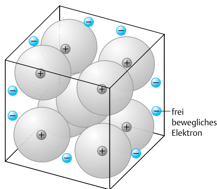
Abb. 1.11 Das Elektronengasmodell
