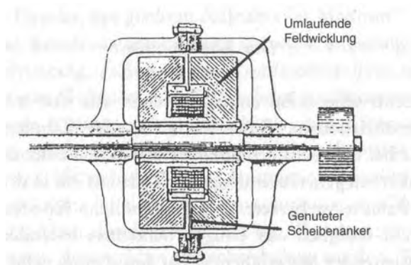
Hochfrequenzdynamo
