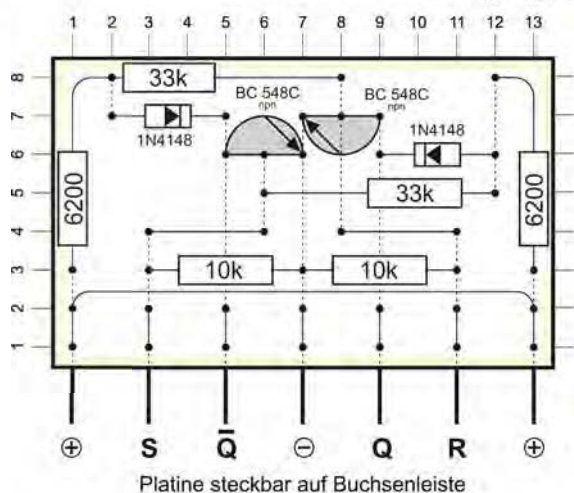
Lochrasterplatine 13 x 8 Punkte mit Streifenaufgabe M = 2 : 1
