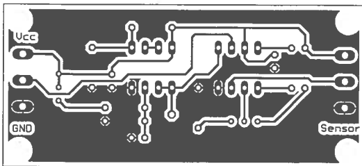
Bild 7: Layoutvorschlag für die Sensorbaugruppe; Abmessungen 69 mm x 31 mm, M 1:1
