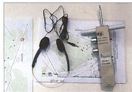
Ein zum Einsatz gekommenes Peilgerät R3500A samt Kartenmaterial Fotos: DL3MSG, DF6OE
