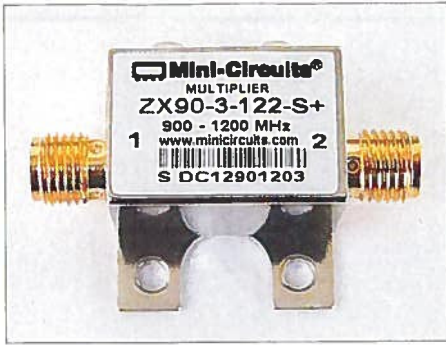
Bild 10: Mini-Circuits-Frequenzverdreifacher vom Typ ZX90-3-122-S im Metallgehäuse mit SMA-Steckverbindern
