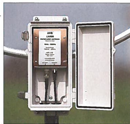
Bild 2: Bei geöffnetem Wetterschutzgehäuse sieht man die Verstärker- und Abstimmeeinheit. Von unten werden das Antennen- und das Steuerkabel geschützt hineingeführt.
