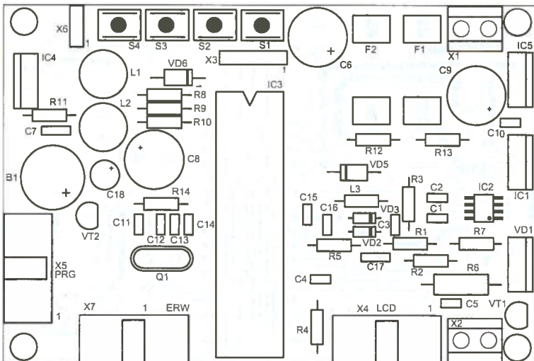
Bild 8: Bestückungsplan der Baugruppe ESS_Z; Abmessungen 100 mm x 67 mm, M 1:1
