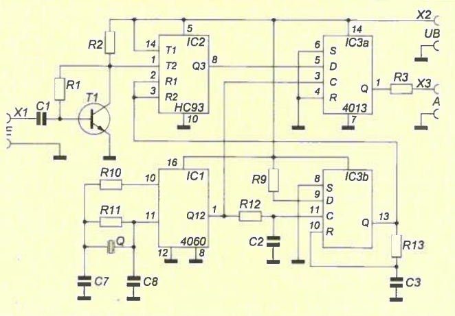
Bild 2: Basis für den Leiterplattenentwurf ist eine mit Anschlussnummern versehene Schaltung, hier das Digitalteil der DAFC aus [3]. Die Form ist zweitrangig – selbst eine Handskizze wäre verwendbar.
