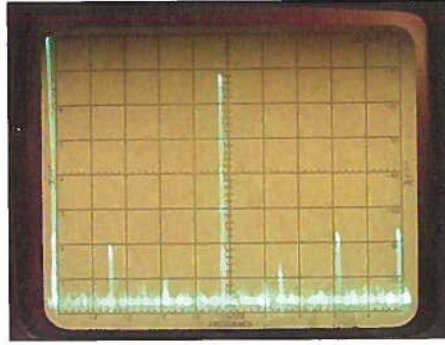
Bild 11: Ausgangssignal des ZX90-3-122-S bei 300-MHz am Eingang; horizontal: 200 MHz/Teilstich, vertikal: 10 dB/Teilstich
