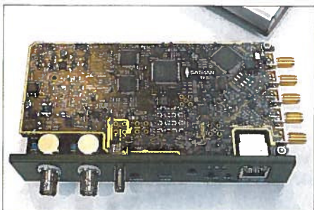
Das „Schweizer Messer“ für SDR: Ein Prototyp des bis in den Gigahertzbereich nutzbaren SDR-Trasceivers TX8M aus Estland
