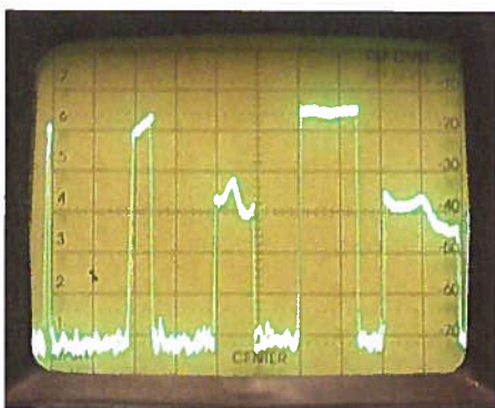
Bild 8: Verdreifachter-Ausgangssignal bei 200 bis 250 MHz am Eingang (Skalierung wie in Bild 3)
