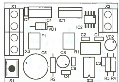
Bild 9: Bestückungsplan der Baugruppe ESS; Abmessungen 50 mm x 35 mm, M 1:1
