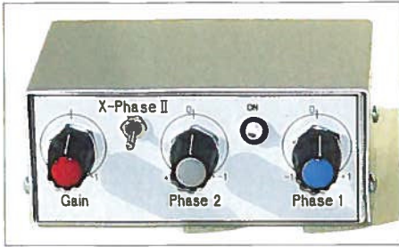
Bild 3: Die fertige X-Phase II mit 14-mm-Spannzangendrehknoepfen; groeere Knoepfe erlauben eine einfachere Bedienung.
