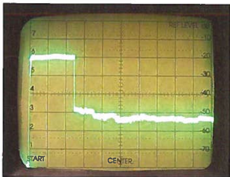
Bild 3: Signal am Ausgang des Wobbeldurchgangs; Skalierung horizontal: 100 MHz/Teilstrich, vertikal: 10 dB/Teilstrich
