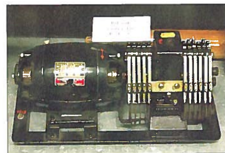
Ruf- und Signalmaschine; diese erzeugte Frei- und Besetztzeichen.
