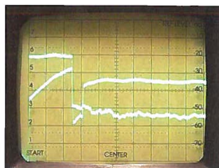
Bild 5: Übereinander gelegte Darstellung des Ein- und Ausgangssignals des Verdreifachers von 130 MHz bis 450 MHz
