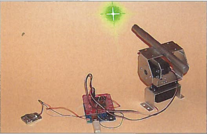
Bild 1: Musteraufbau der Elektronik für den Fingerhakeltrainer mit (v. l. n. r.) Kraftsensor, Arduino-Board und Servomotor mit Laser Foto: Sander
