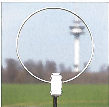
Bild 1: Rahmen und Verstärkergehäuse sind wetterfest für den Außenbetrieb konzipiert.
