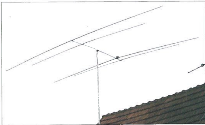
Bild 1: Ansicht des von ON8DM aufgebauten 2-Element-Beams für die Bänder 10 m und 15 m
