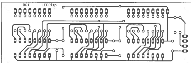
Bild 9: Lötseite der Leiterkarte zur LED- Ansteuerung; Abmessungen 98,5 mm x 32 mm, M 1:1
