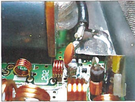
Bild 5: Blick auf den angelöteten Keramik-kondensator
