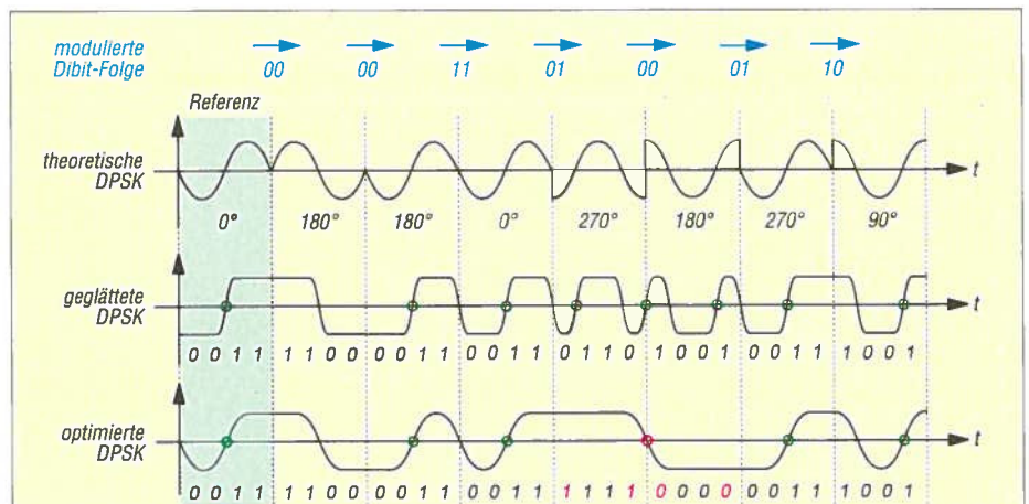
Bild 4: Beispiel zur 4-DPSK einer Dibit-Folge; zu erkennen ist der Unterschied zwischen Standard und optimierter Codierung.
