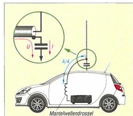
Bild 3: Wenn sich die Mantelwellendrossel nicht unmittelbar am Antennenfußpunkt befindet, wird das erste Stück des Speisekabels zum Teil der Antenne. Der Strom dieses „Radials“ erzeugt am Antennenfußpunkt einen Spannungsabfall, der in das Antennenkabel eingekoppelt wird – trotz Mantelwellendrossel.
