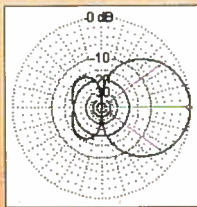
Richtstrahler
