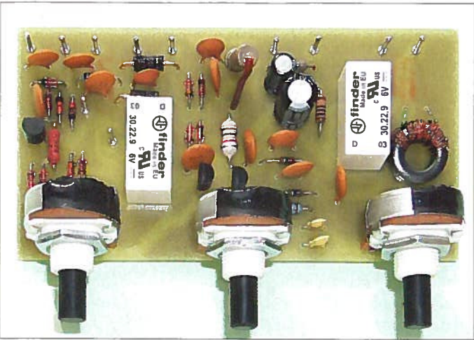
Bild 6: Blick auf die vollständig bestückte Platine; rechts über dem Potenziometer ist der Übertrager Ü1 zu erkennen.
