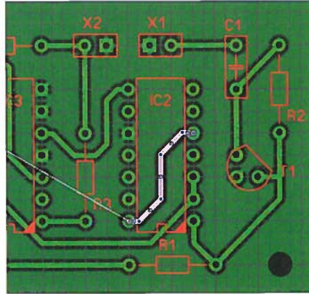
Bild 6: In der Regel ist immer das manuelle Verändern der Leiterbahnen notwendig.
