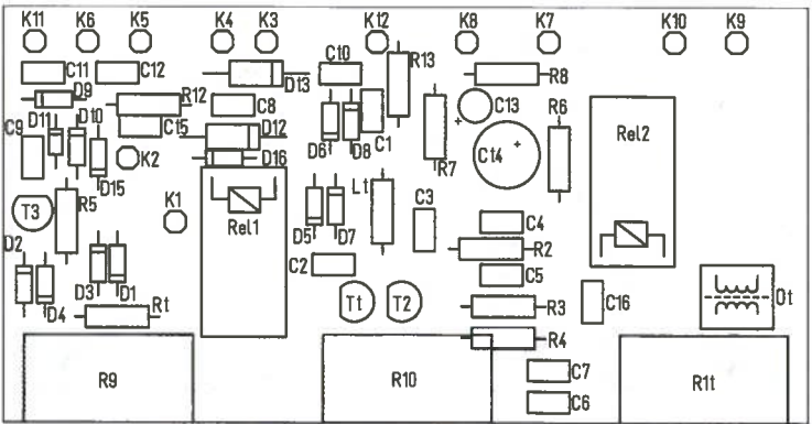
Bild 7: Bestückungsplan der Platine; Abmessungen 97,5 mm x 50 mm, M 1:1
