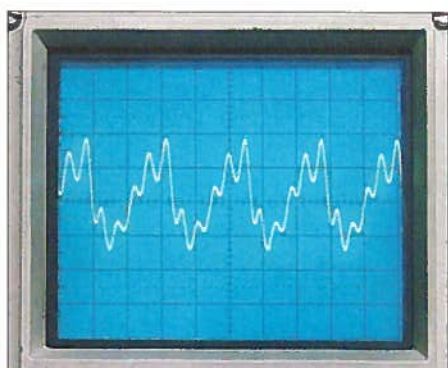
Bild 9: Mit dem Oszilloskop am Ausgang des RMK-3-92 gemessenes Signal bei 130 MHz am Eingang
