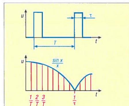
Bild 5: Ein „Lattenzaun“ im Frequenzbereich entsteht im Allgemeinen aus schmalen, steilen Impulsen. Oben sind diese im Zeitbereich zu sehen, unten das von ihnen erzeugte Spektrum im Frequenzbereich.
