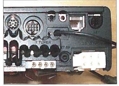
Bild 7: Teil der Rückseite des IC-706 mit Kabelführung durch ein vorhandenes Loch
