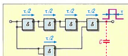
Bild 6: Eine häufige Quelle für den „Lattenzaun“ im Frequenzbereich sind logische Gatternetzwerke. Ein Kondensator geringer Kapazität (rot eingezeichnet) sorgt hier für Ruhe, ohne die Flanken unzulässig zu verschleifen.
