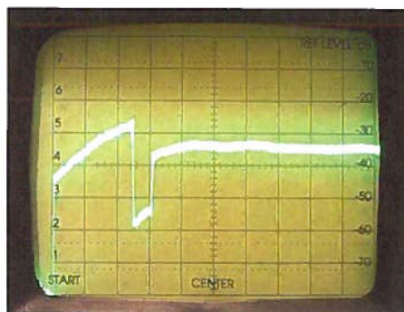
Bild 4: Verdreifachter-Ausgangssignal bei Ansteuerung mit Signal gemäß Bild 3 (Darstellung mit gleicher Skalierung)
