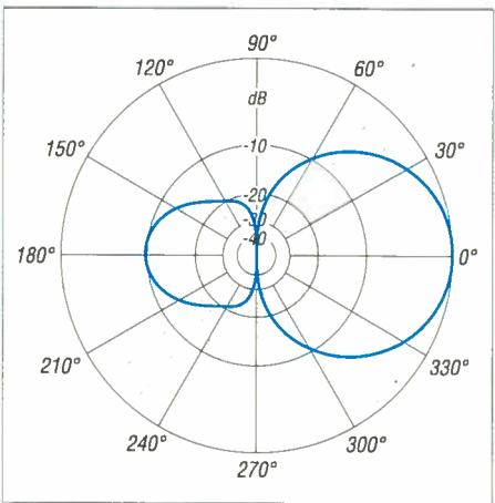
Bild 4: Simuliertes horizontales Freiraumdiagramm für 21,2 MHz
