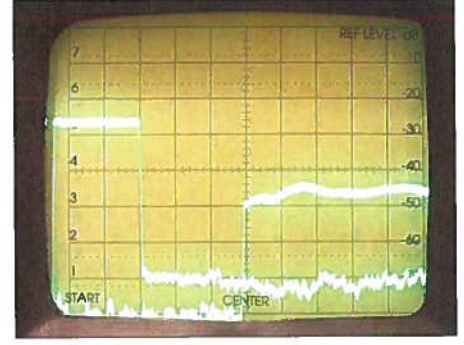
Bild 12: Ein- und Ausgangssignale bei 270 MHz bis 500 MHz am Eingang; horizontal: 100 MHz/Teilstich, vertikal: 10 dB/Teilstich
