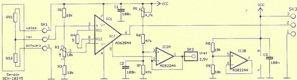
Bild 3: Schaltung der Sensorbaugruppe, in der ein Instrumentationsverstärker, hier der AD620, zum Einsatz kommt
