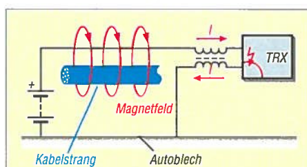
Bild 4: Magnetfelder induzieren in Leiterschleifen symmetrische Ströme, die von einer gemeinsamen Mantelwellendrossel nicht unterdrückt werden können. Deshalb sollte man möglichst jeden Leiter einzeln verdrosseln.
