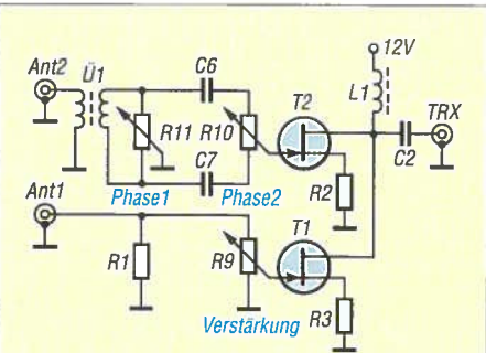
Bild 2: Prinzipschaltung der X-Phase II; an der Buchse Ant1 ist die Haupt- und an der Buchse Ant2 die Hilfsantenne angeschlossen.
