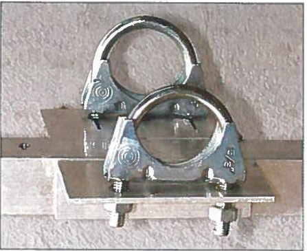
Bild 5: Die Befestigung des 2-Element-Beams am Mast erfolgt mit zwei Aluminiumwinkeln sowie Auspuff- und dazu passenden Krallenschellen.
