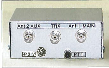
Bild 4: Gehaeuserueckseite des X-Phase II, hier mit BNC-Buchsen versehen; alternativ sind auch PL-Buchsen einsetzbar.
