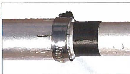
Bild 8: Nach dem Lösen der Schellen lassen sich die Elementabschnitte zum Abgleich ineinander schieben.
