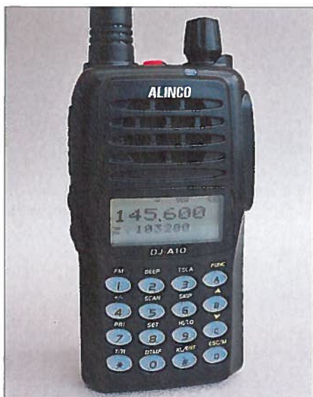
Bild 1: Die Tastatur wird bei Bedienung hellweiß durchleuchtet, das Display wahlweise bernsteingelb, violett oder blau beleuchtet.
