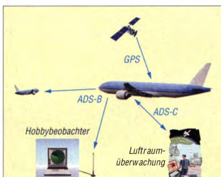
Bild 1: Flugzeuge bestimmen ihre Position mittels GPS und senden diese sowie weitere Fluginformationen per ADS-B ungerichtet auf 1090 MHz. ADS-C dient für bidirektionale Verbindungen mit der Flugkontrolle.
