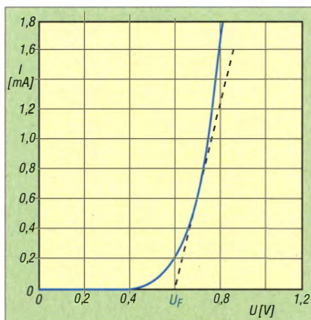
Bild 5: Kennlinie einer Silizium-Diode 1N4148; die im Original für D7 verwendet SAY30 besitzt ähnliche Werte.
