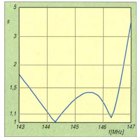
Bild 18: Das simulierte SWV der OWL-Yagi von 143 MHz bis 147 MHz sieht so ähnlich aus wie die Anpassungskurve eines Bandfilters.
