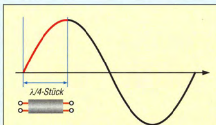
Bild 13: Ein Stück Übertragungsleitung mit der entsprechenden charakteristischen Impedanz und der geometrischen Länge, die exakt einem Viertel der zu übertragenden Wellenlänge entspricht, transformiert die Widerstandsverhältnisse so, dass die Last als optimal angepasst erscheint.
