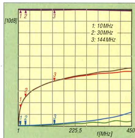
Bild 4: Messergebnisse für Schaltstellungen 1/2 der „KW- und 144-MHz-Version“; Einfügedämpfung a_D [dB] (lila/schwarz, etwa deckungsgleich), Übersprechdämpfung a_U [dB] (braun/rot), SWV (blau/grün)
