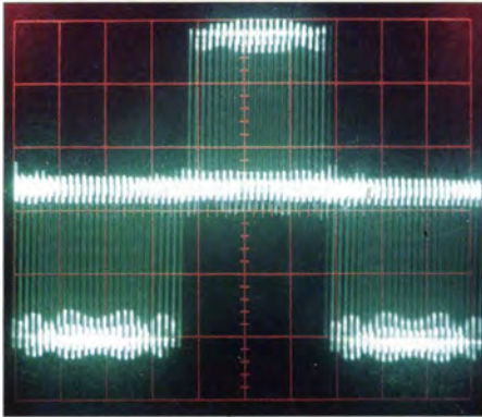
Bild 3: Oszillogramm eines Sinussignals an den Ausgangspins SP+ und SP- des Sprachspeicher-IC
