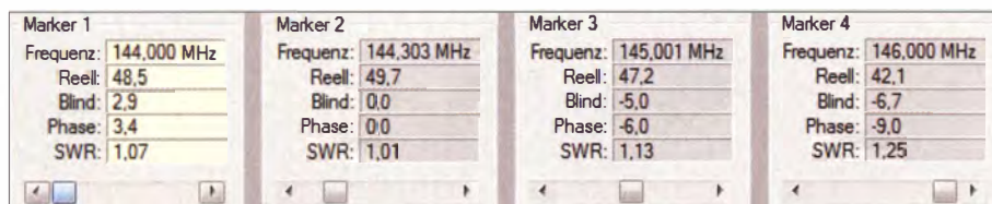
Bild 17: Die exzellente Anpassung der OWM-Yagi im kompletten 2-m-Band, hier zusätzlich mit Angabe von Wirk- und Blindanteil der Impedanz
