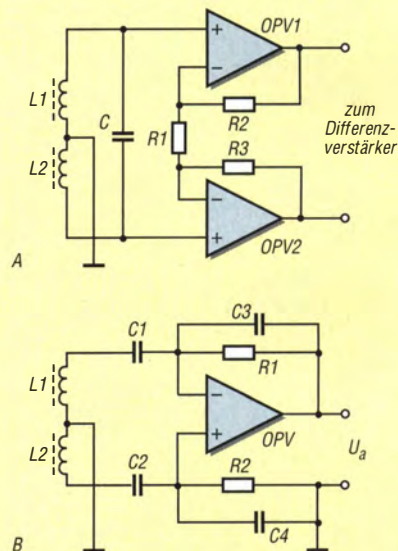
Bild 26: Ankopplung des symmetrischen Parallelschwingkreises an eine Instrumentationsverstärker-Eingangsstufe (oben) sowie Ankopplung eines symmetrischen Serienschwingkreises an einen Differenzverstärker (unten)
