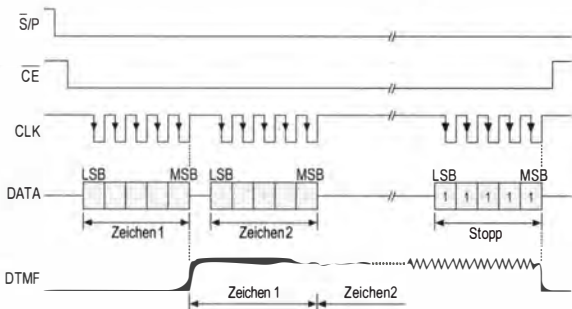
Bild 4: Steuersignale im seriellen Modus
