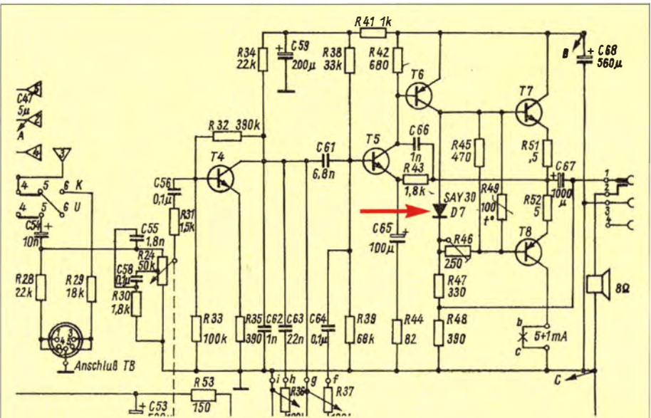
Bild 3: Schaltungsausschnitt der NF-Stufe des Stern Automatik 1421; die zur Beseitigung der Verzerrungen erforderliche Tunneldiode muss in Reihe mit der Diode D7 eingelötet werden, sodass sich Anode und Katode gegenüberstehen.
