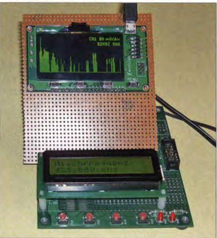
Bild 1: Versuchsaufbau des Spektrumskops mit dem auf einer Universalplatine aufgesetzten Oszilloskopmodul Xprotolab und einem Staver24-Board als Steuerung
