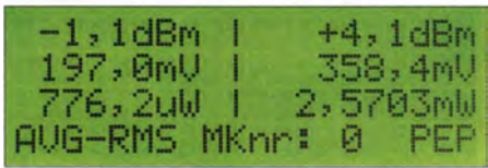
Bild 22: Signalpegel meines Zweitongenerators; dieser hat einen IMA3 von etwa 90 dB.
