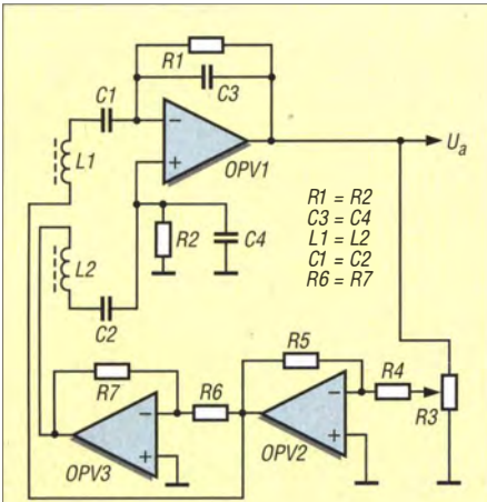
Bild 27: Prinzipschaltung zur Entdämpfung eines symmetrisch angeordneten Serienschwingkreises
