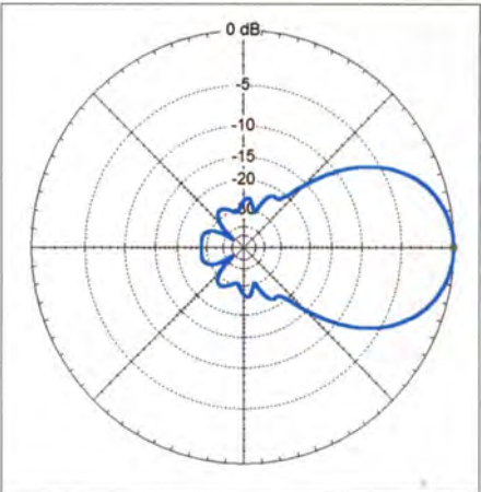
Bild 9: Simuliertes vertikales Richtdiagramm der 8-Element-OWL-Yagi im Freiraum (0 dB ≙ 11,0 dBd)
