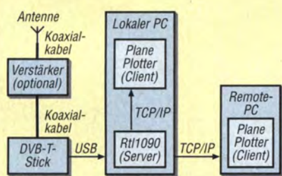
Bild 2: Das Empfangssignal gelangt von der Antenne über den DVB-T-Stick zum PC. Dort erfolgen per Software die Verarbeitung und grafische Darstellung.
