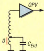
Bild 25: Der Spulenanschluss der oberen Lage liegt auf Masse und der rot markierte, mit 0 gekennzeichnete Wicklungsteil somit an der Spulenoberfläche. Er bildet C_{\text{Erd}} aus.
