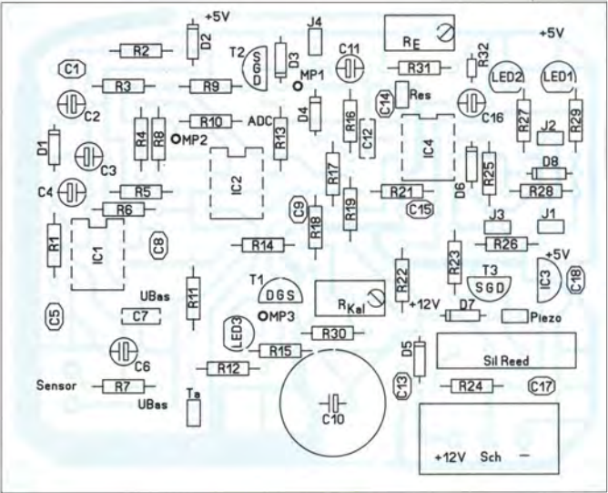
Bild 6: Bestückungsplan der nur mit bedrahteten Bauteilen bestückten Leiterplatte des Drucksensors
