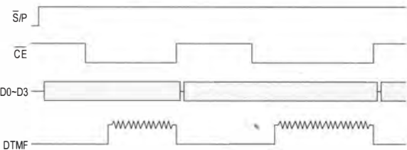
Bild 5: Steuersignale im parallelen Modus
