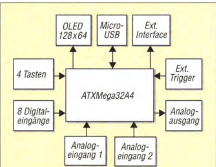
Bild 2: Blockschaltbild der identischen Oszilloskopmodule
