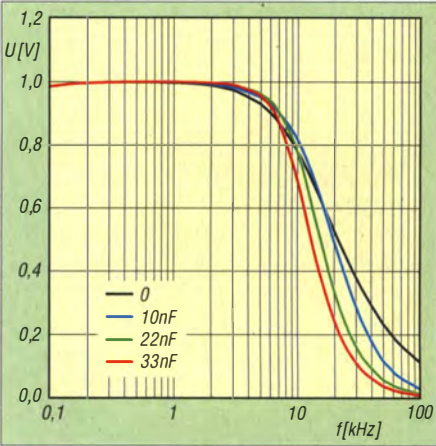
Bild 7: Frequenzgang des Sprachspeichers bei Wiedergabe in Abhängigkeit von C31
