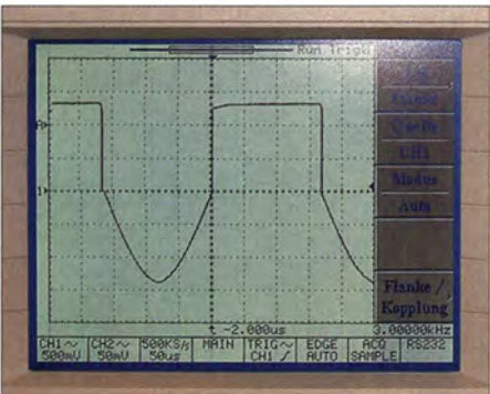
Bild 2: Messkurve des fehlerhaften Signals bei großen Eingangsspannungen
