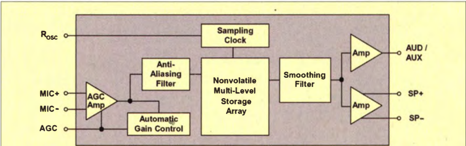
Bild 2: Auszug aus dem Blockschaltbild des Datenblatts mit dem Analogteil des Sprachspeicher-IC ISD1700; der Verstärker für die Ausgänge SP+ und SP- besteht nur aus zwei zeitgesteuerten Schaltern.
