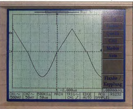
Bild 1: Messkurve des fehlerhaften Signals bei kleinen Eingangsspannungen, aufgenommen mit einem Voltcraft DSO 6150S
