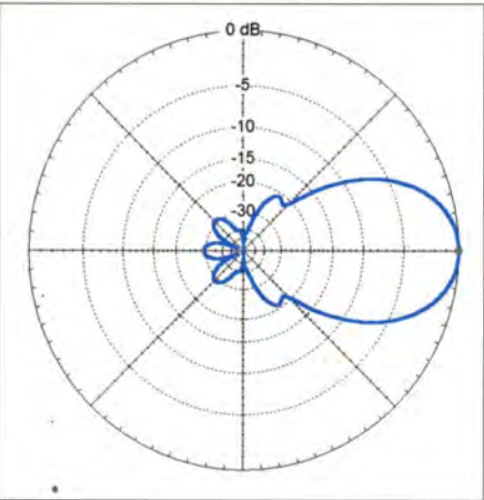
Bild 11: Simuliertes horizontales Richtdiagramm der 8-Element-OWM-Yagi im Freiraum (0 dB \hat{=} 11,07 dBd)
