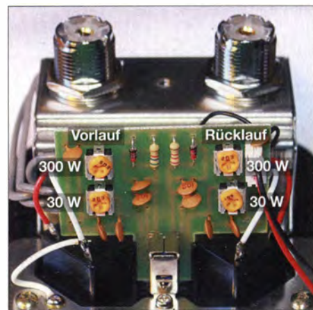
Bild 3: Gleichspannungsplatine für die Anzeige; die Funktion der einzelnen Trimpotenzimeter ist in Weiß eingetragen.
