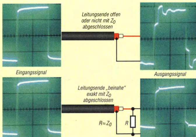
Bild 12: Wenn das Ende der Übertragungsleitung nicht mit dem richtigen Wellenwiderstand abgeschlossen ist (Fehlanpassung), können Reflexionen die übertragenen Signale überlagern und damit verzerren. Bei möglichst impedanzrichtiger Anpassung lassen sich Leitungsreflexionen vermeiden.
