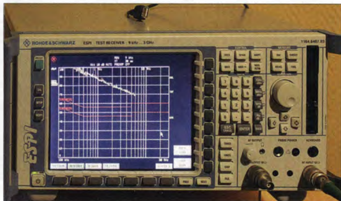
Bild 4: Störpotenzial des Schaltnetzteils eines Mobiltelefon- Ladegeräts
