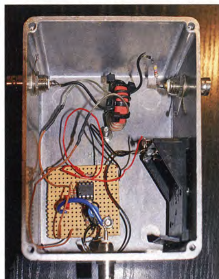
Bild 3: Experimentalaufbau eines Vorverstärkers für Loop-Antennen nach [1]; zwischen den Anschlussbuchsen der Antennenschleife liegen das Anpassglied (Ringkern) für den Vorverstärker und in Serie damit der Schluckwiderstand. Foto: OE5CWL
