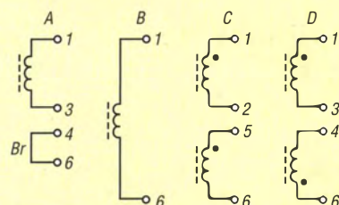
Bild 21: Varianten der Anschaltung von Induktionsspulen an das Experimentiermodul nach Bild 20; für Ausführung D sind zwei Kreiskondensatoren erforderlich, bei C und D ist der Spulenwickelsinn zu beachten.
