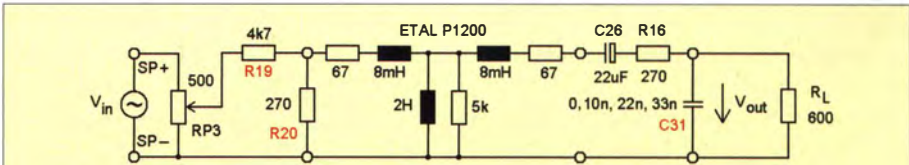
Bild 6: Schaltbild zur Schaltungssimulation; die rot dargestellten Bauteile sind neu hinzugekommen.
