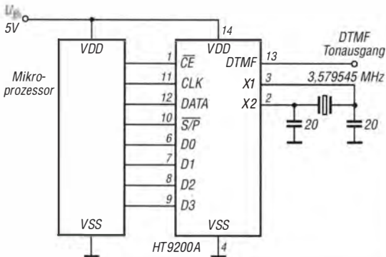
Bild 6: DTMF-Tongenerator mit einem HT9200B und wahlweise paralleler oder serieller Ansteuerung
