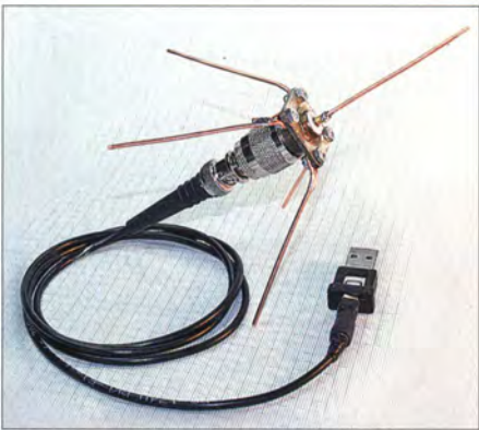
Bild 3: Die minimale Hardware-Ausstattung besteht aus einer Groundplane-Antenne, die über ein kurzes Kabel mit einem DVB-T-Empfangsstift für die USB-Schnittstelle verbunden ist.
