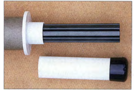
Bild 31: Verlängerung der Induktionsspule durch zusätzliche Rohrstücke; die Gesamtlänge des Rohres beträgt 86 cm. Angereicht sind vier Stabkerne mit je 30 mm Durchmesser und 200 mm Länge. Die Spule hat 100 000 Windungen (CuL, 0,18 mm).
