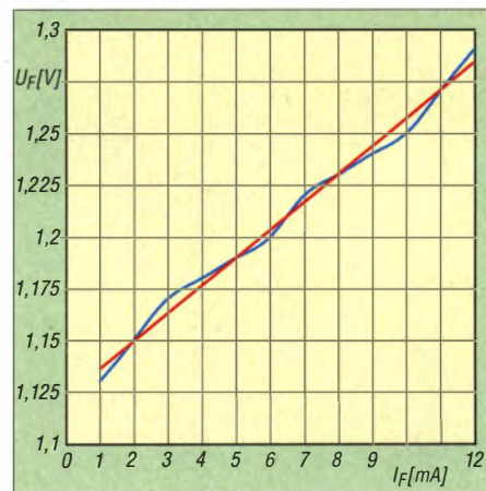
Bild 1: Gemessene (blau) und idealisierte Kennlinie (rot) der LED im Optokoppler
