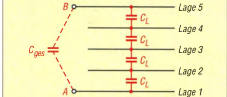
Bild 24: Bei mehrlagigen Spulen entsteht eine Reihenschaltung der Lagenkapazität; C_{ges} ist die resultierende Ersatzkapazität.
