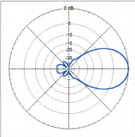
Bild 8: Simuliertes horizontales Richtdiagramm der 8-Element-OWL-Yagi im Freiraum (0 dB ≙ 11,0 dBd)
