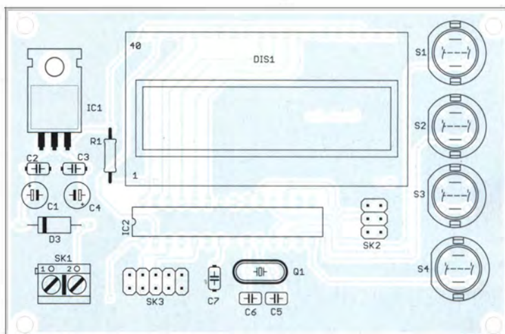
Bild 8: Bestückungsplan der nur mit bedrahteten Bauteilen aufgebauten Controllerbaugruppe; Abmessungen 98 mm × 63 mm, M 1:1
