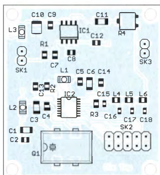
Bild 7: Bestückungsplan der vollständig mit SMD-Bauteilen aufgebauten Mischerleiterplatte; Abmessungen 47 mm × 44 mm, M 1:1
