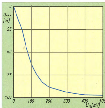
Bild 10: Regelkennlinie von T2 in Abhängigkeit von der Regelspannung U_R
