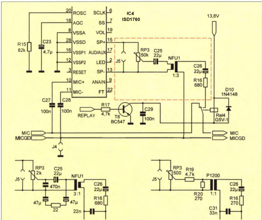
Bild 4: Auszug aus dem Originalschaltplan mit allen für den Sprachspeicher wichtigen Teilen (oben rot gestrichelt umrahmt), Modifikation unter Verwendung des Originalübertragers (unten links), Umbau mit dem NF-Übertrager P1200 (unten rechts)
