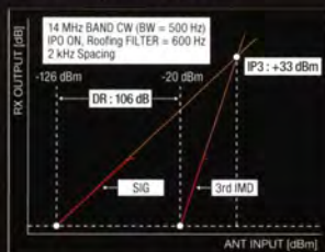
Dynamikbereich 3. Ordnung/IP3
