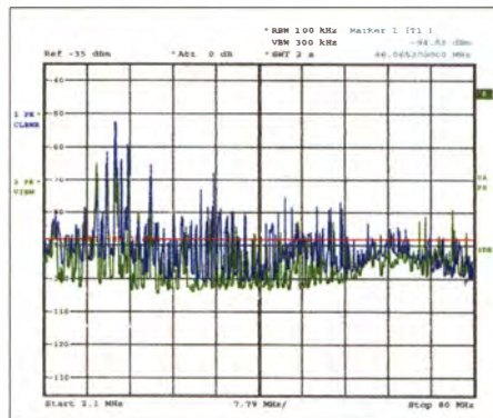
Bild 2: Spektrum nach Beseitigung der Störung; nur leichte Spratzen sind noch da.
