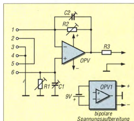
Bild 20: Prinzipschaltung des Experimentiermoduls in Bild 1 (vorige Ausgabe); es lassen sich Induktionsspulen auf unterschiedliche Weise anschließen (Bild 21); die Erweiterung zu Reihenschwingkreisen ist möglich.
