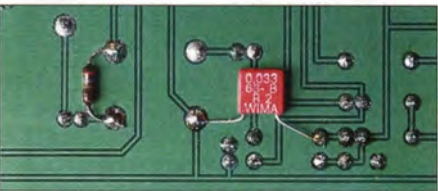
Bild 8: Nur zwei Bauteile sind auf der Platinenrückseite zu ergänzen.
