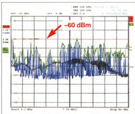
Bild 1: Breitbandiges Störspektrum; Start 2,1 MHz, Stopp 80 MHz, 5 dB/Div
