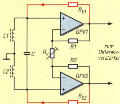
Bild 28: Prinzipschaltung zur Entdämpfung eines symmetrisch angeordneten Parallelschwingkreises
